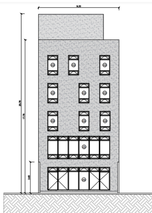
CORTE GG - VISTA CONTRAFRENTE
