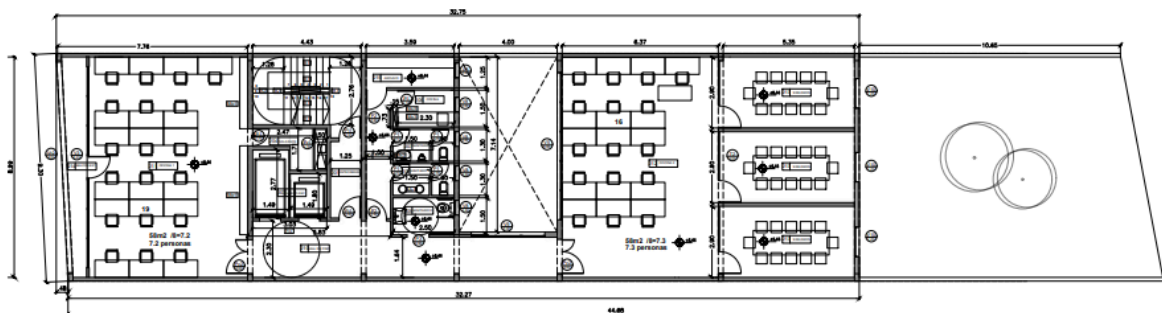
D E F G Planta 2º piso
