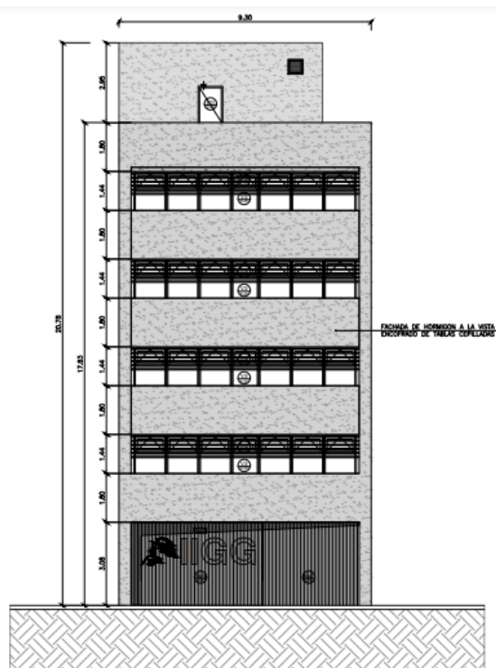
VISTA ESTE FRENTE
